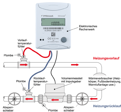
Schematischer Aufbau eines elektronischen Wärmehählers, hier in Ausführung eines Splittgerätes mit voneinander getrennten Einzelkomponenten.
